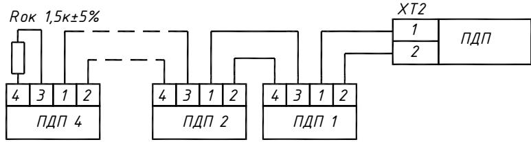
Рис.2.3. Подключение ПДП.
