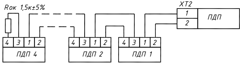
Рис.2.3. Подключение ПДП.
